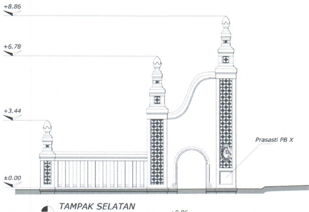
Gambar 1. Gambar Gapura Madegondo tampak selatan (Sumber: Dinas Pendidikan dan Kebudayaan Kabupaten Sukoharjo, 2023)
