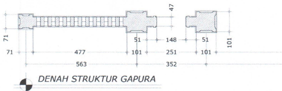
Gambar 3. Gambar denah Struktur Gapura Madegondo (Sumber: Dinas Pendidikan dan Kebudayaan Kabupaten Sukoharjo, 2023)
