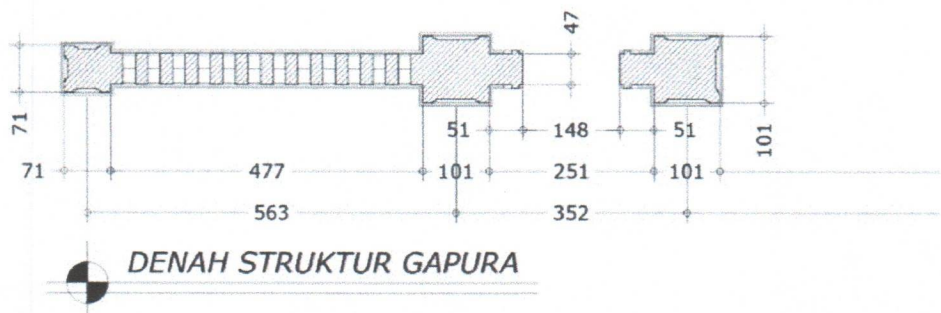
Gambar 3. Gambar Denah Struktur Gapura Grogol (Sumber: Dinas Pendidikan dan Kebudayaan Kabupaten Sukoharjo, 2023)
