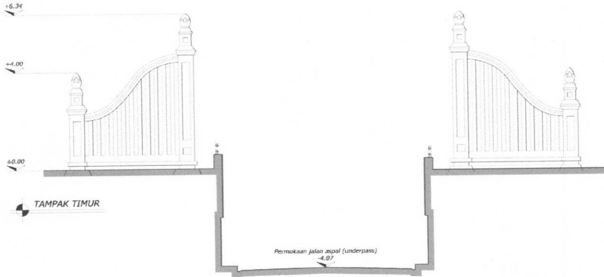
Gambar 1. Gambar Gapura Makamhaji tampak timur (Sumber: Dinas Pendidikan dan Kebudayaan Kabupaten Sukoharjo, 2023)
