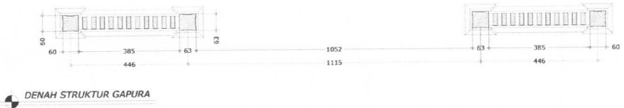
Gambar 3. Gambar denah Struktur Gapura Makamhaji (Sumber: Dinas Pendidikan dan Kebudayaan Kabupaten Sukoharjo, 2023)
