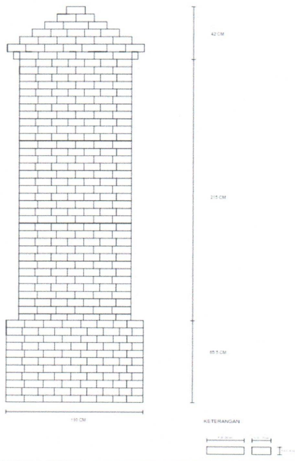
Gambar 7.1. Gambar Potongan Struktur Pagar Dalem Singapuran (Sumber:Dinas Pendidikan dan Kebudayaan Kabupaten Sukoharjo, 2021)
